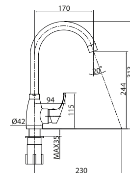
Смеситель для кухни
