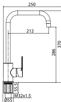
Смеситель для кухни
