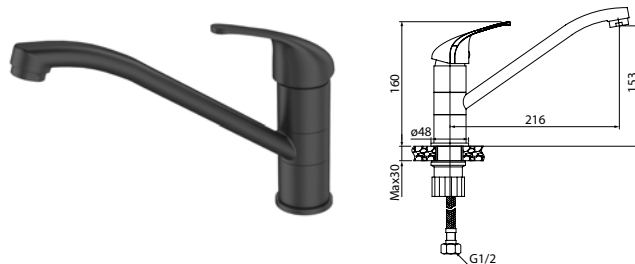
Смеситель для кухни
