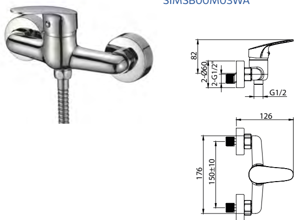
Смеситель для душа
