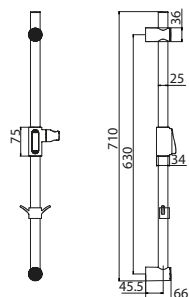
Стойка для душа ILS70COM17
