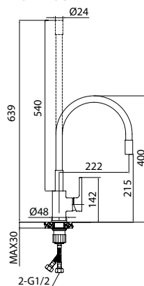
Смеситель для кухни с гибким изливом
