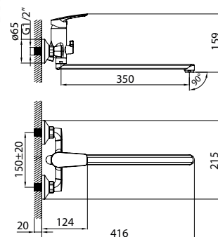
Смеситель для ванны с длинным изливом
