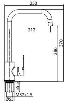
Смеситель для кухни
