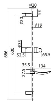
Стойка для душа
