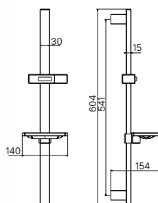
Стойка для душа ILS60BSM17
