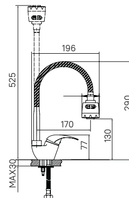
Смеситель для кухни с гибким изливом и душевой насадкой
