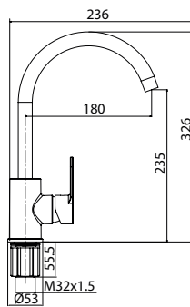
Смеситель для кухни
