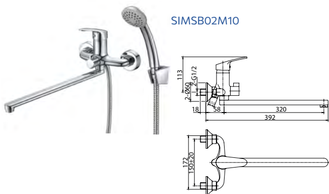
Смеситель для ванны с длинным изливом
