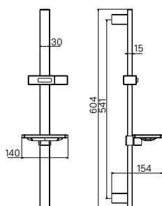
Стойка для душа ILS60CSM17
