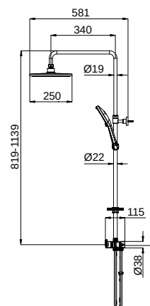
Душевой гарнитур с тропической лейкой
