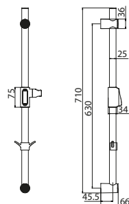
Стойка для душа ILS70BOM17
